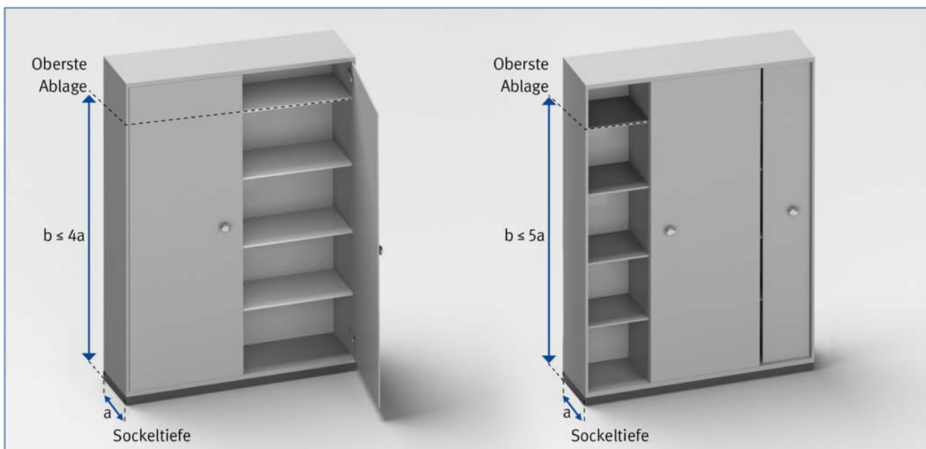
Abb. 37 Verhältnis der Sockeltiefe zur Höhe der obersten Ablage
